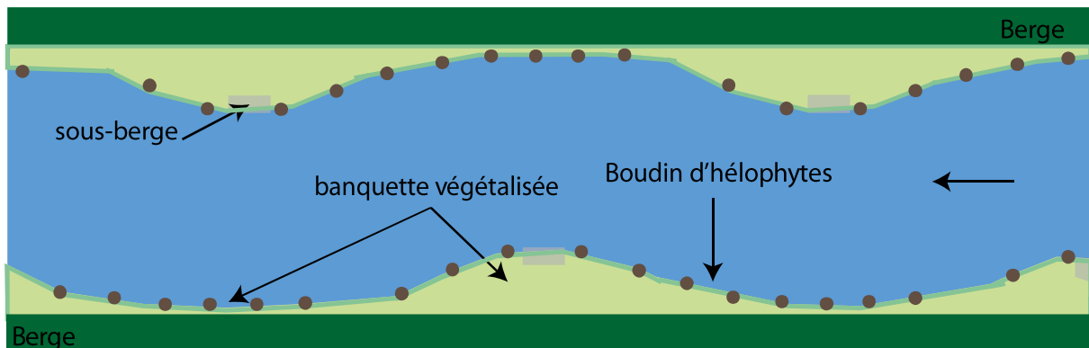
Schéma simplifié de l'aménagement du secteur aval
